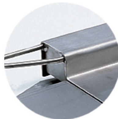
Détail du profilé conçu pour faciliter le nettoyage de la plate forme
